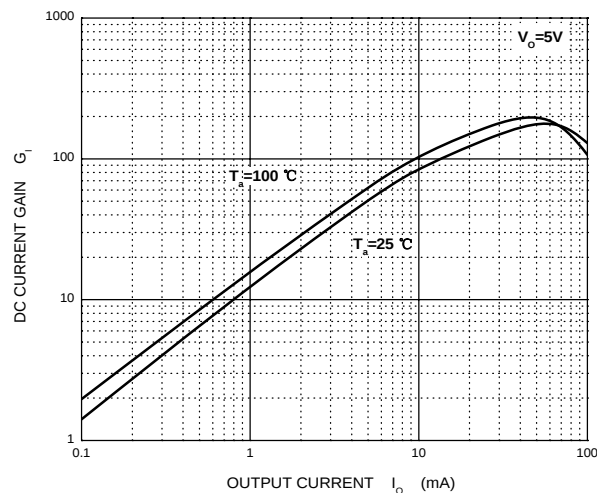
G_I - I_O
