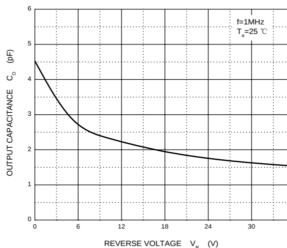
C_O - V_R
